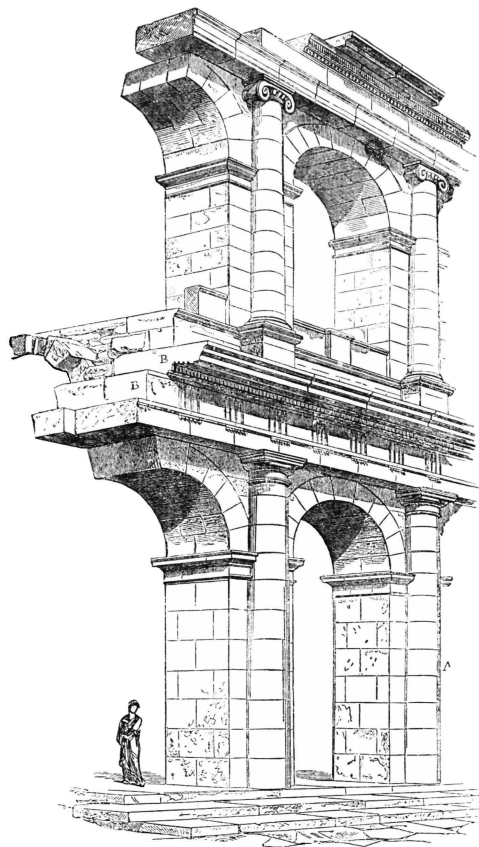
Fig. 2. Dal teatro di Marcello a Roma (secondo Viollet-le-Duc).
