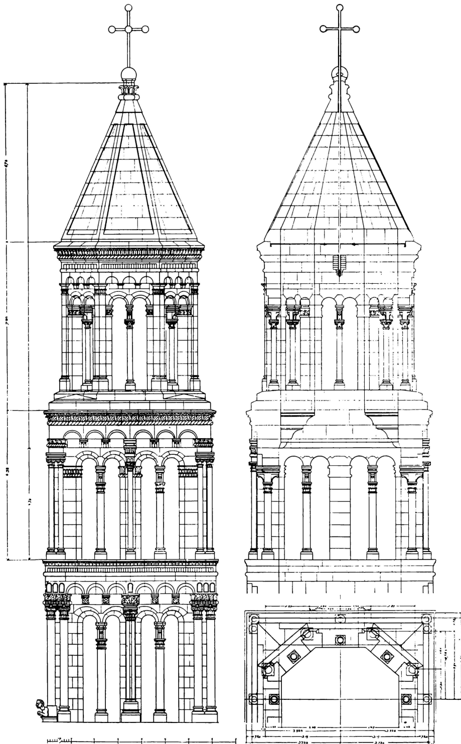
Alzato del IV. V. e VI. Ordine del Campanile secondo il progetto Förster.
