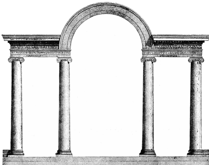
Fig. 3. Acquedotto di Adriano in Atene (secondo Stuart e Revett).
